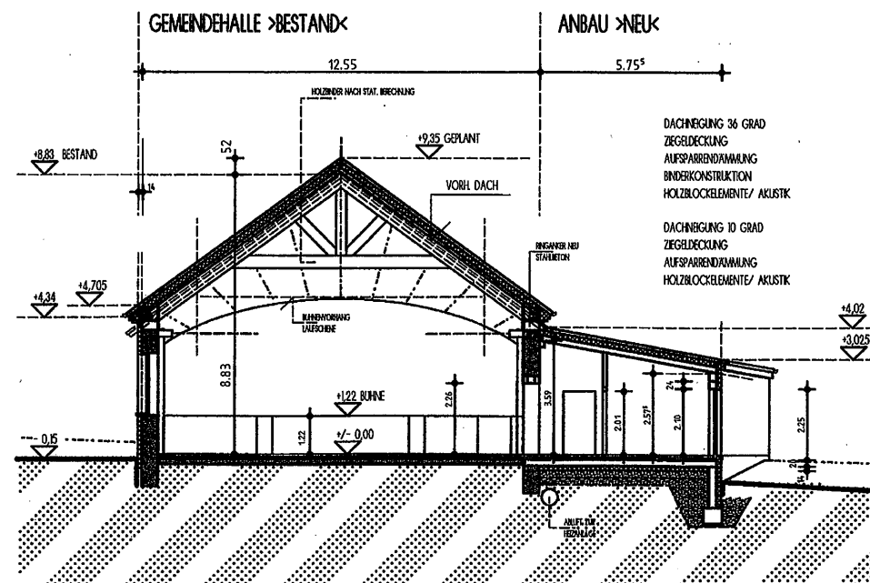
SCHNITT A-A
